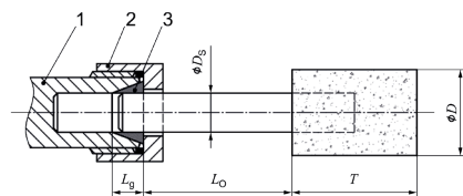
Obrázek 1 - Délka upnutí sklíčidla a kleštiny
