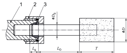
Figura 1 - Longitud de sujeción del mandril y mordaza
