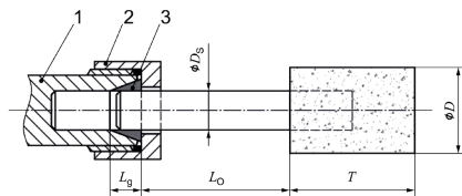
Εικόνα 1 — Μήκος τοποθέτησης εργαλειοδέτη και κόλετ
