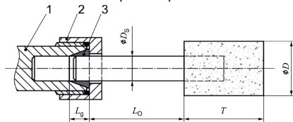
Kuva 1 – Kiristinistukan ja kiristyspihdin kiinnityspituus
