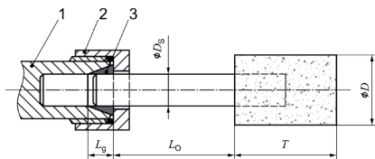
Afbeelding 1 - Spanlengte van de spankop en spantang
