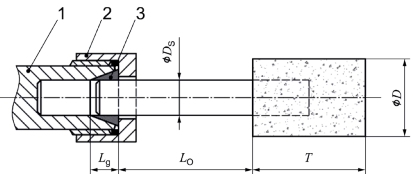
Obrázok 1 - Upínacia dĺžka upínacieho puzdra a upínacích klieští
