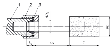
Afb. 1 - spændepatronens fastspændingslængde og spændetang
